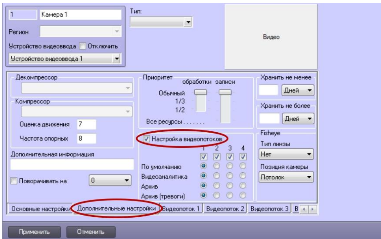
Рис. 1. Включение многопоточности.
