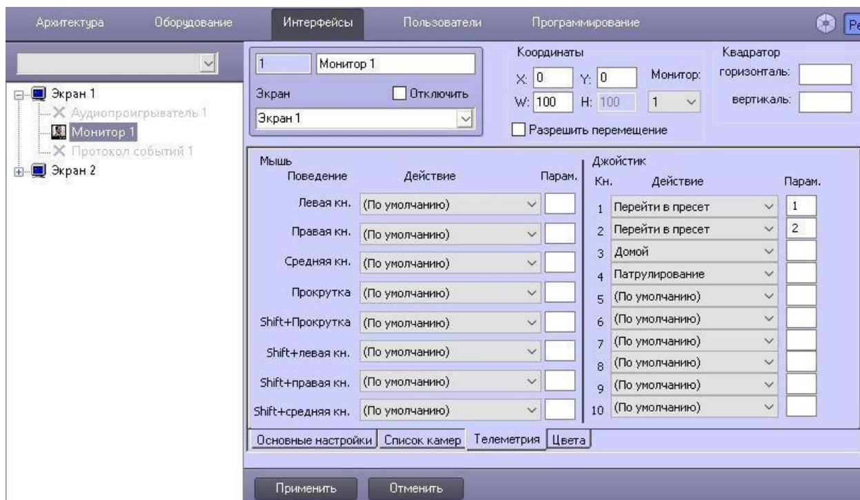
Рис. 2 Настройка горячих клавиш.
